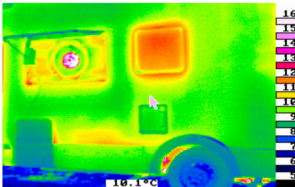
Abbildung 12-2: Thermographie und Dichtheitsprüfung mittels Blowerdoor-Verfahren
