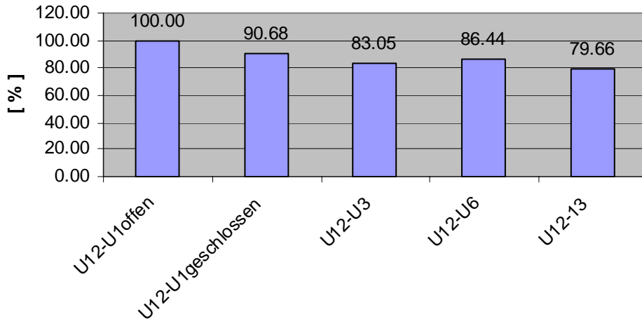
Diagramm 3: Beispiel der Untersuchungen - Darstellung der energetischen Verbräuche in Abhängigkeit von den Veränderungen am Wohnmobil.
