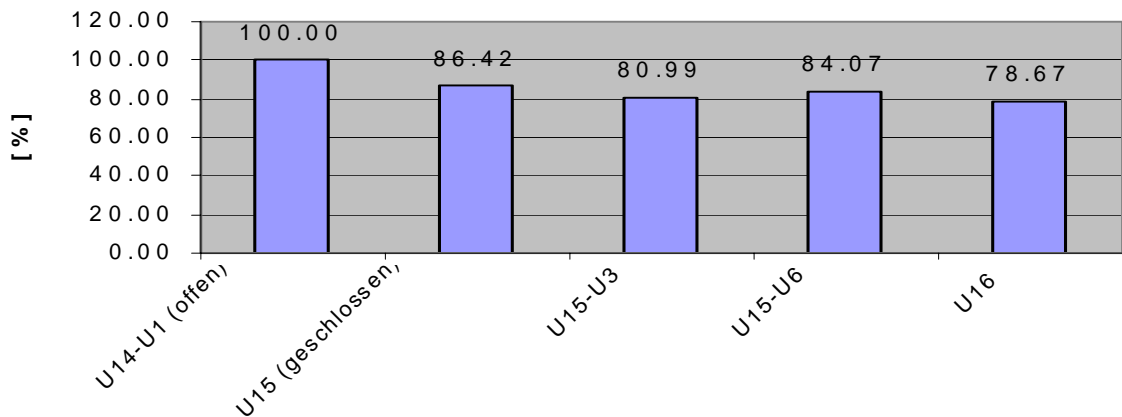
Diagramm 4: Beispiel der Untersuchungen - Darstellung der energetischen Veränderungen in Abhängigkeit von den Veränderungen am Wohnmobil
