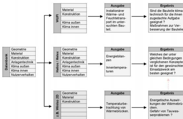
Diagramm 3: Struktur des Programmeinsatzes
