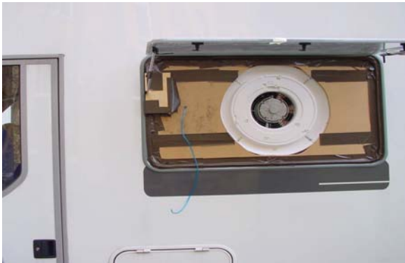
Abbildung 12-2: Anordnung des Blowerdoor Gebläses
