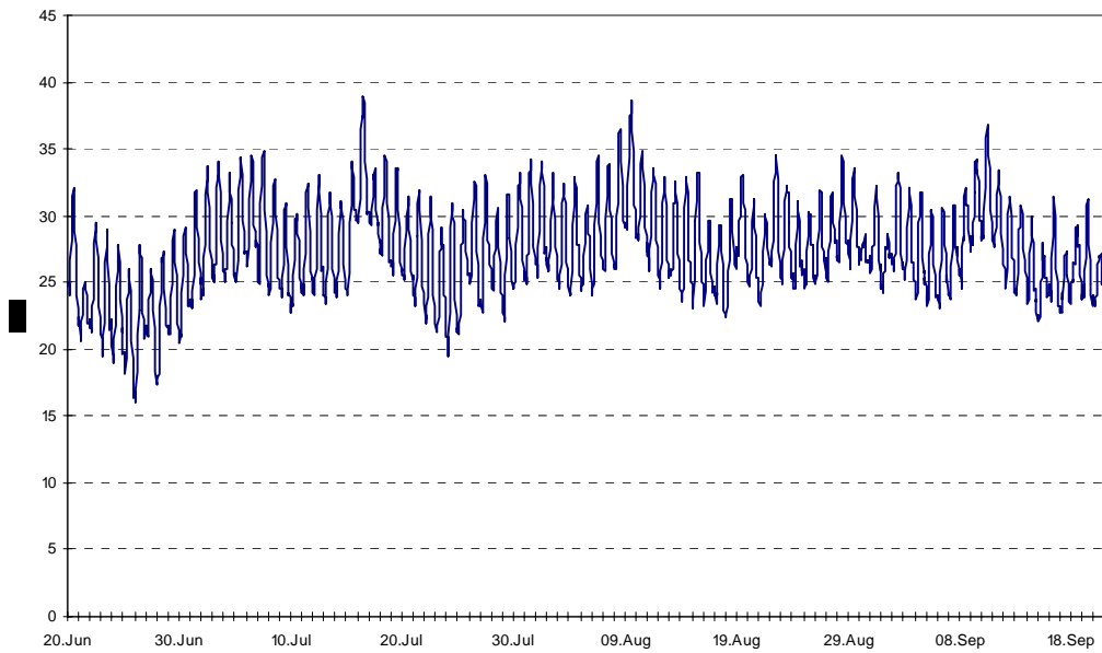
Diagramm 11: Verlauf der Außentemperatur im Untersuchungszeitraum Winter - Almeria-Spanien
