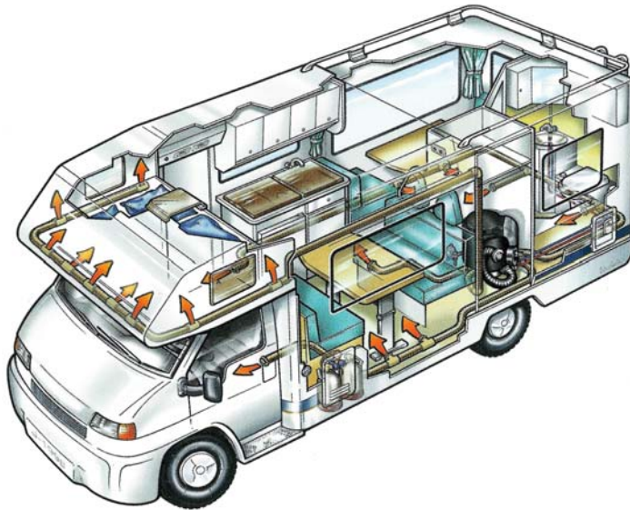
Abbildung 5: Luft-Energieverteilungssystem in einem Wohnmobil
