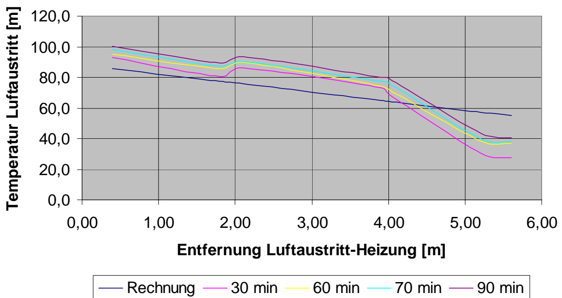
Diagramm 1: Abhängigkeit der Austrittslufttemperatur von der Entfernung vom Heizgerät
