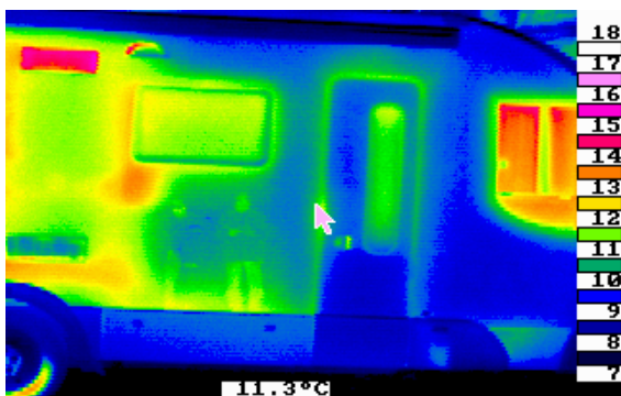
Abbildung 7 Beispiel -Thermografie des Serienzustandes - Beifahrerseite ohne Innenüberdruck
