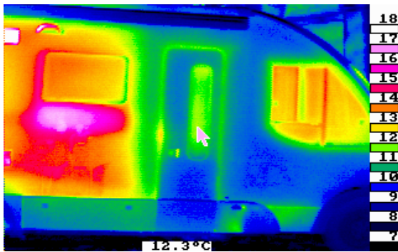
Abbildung 7 Beispiel -Thermografie des Serienzustandes - Konstanter Überdruck im Innenraum von 50 Pascal
