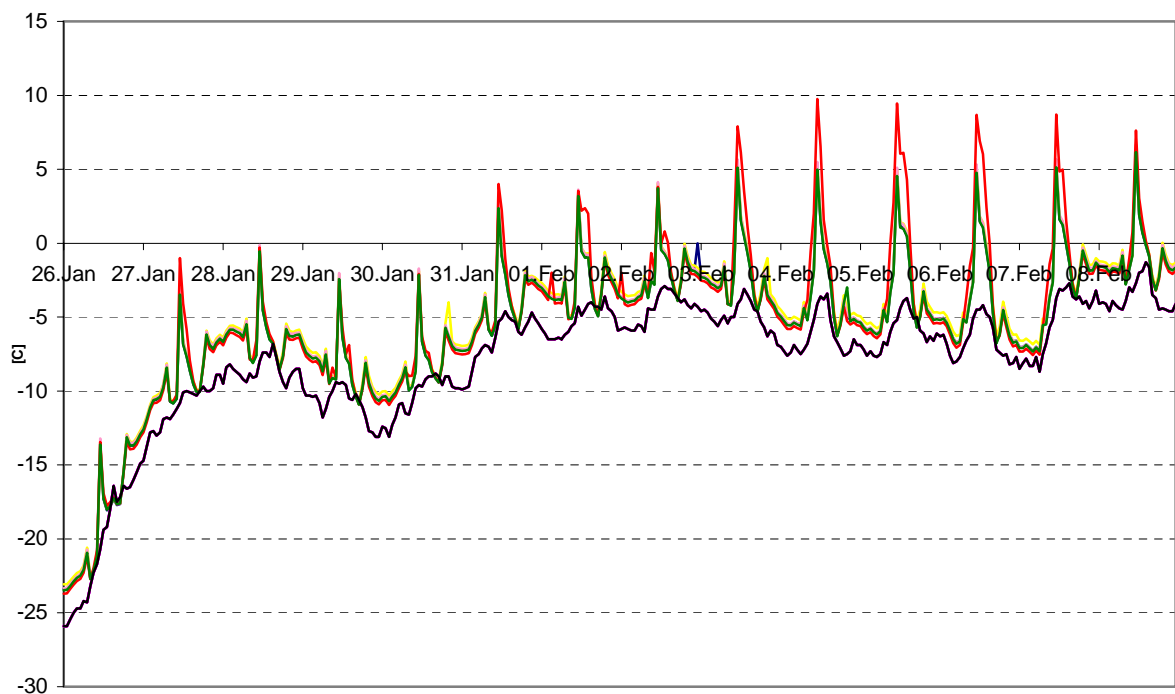
Diagramm 14: Beispiel der Untersuchungen - Innentemperaturen in Abhängigkeit der Wärmedurchlasswiderstände der Außenbauteile;
