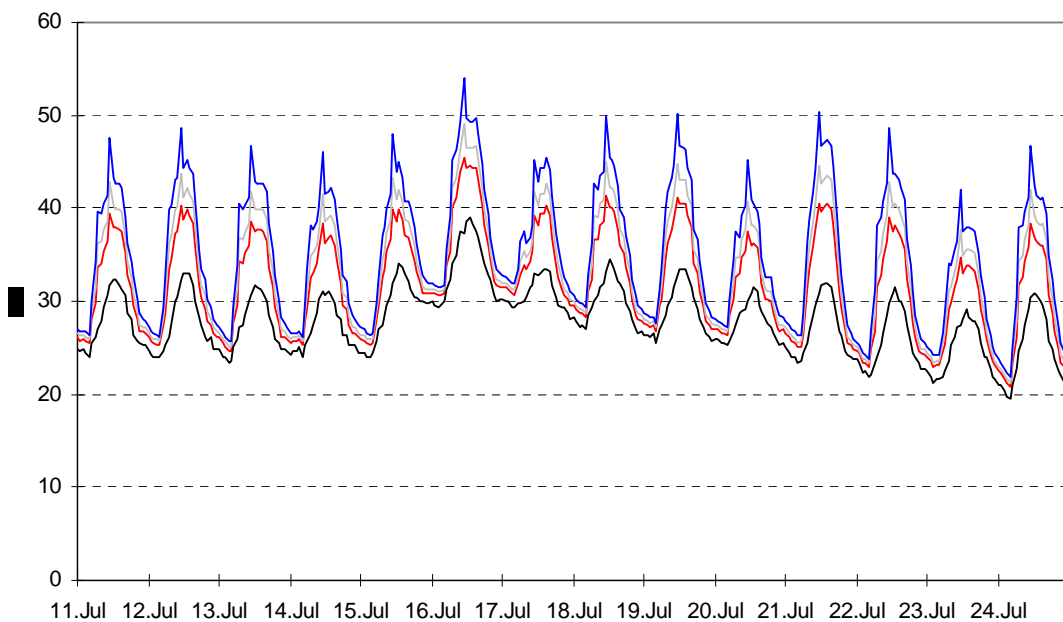
Diagramm 12: Beispiel zu den Untersuchungen - Innentemperaturen in Abhängigkeit der Luftwechsella- ten; LW = 1,5 – blau; LW = 5,0 – grau; LW = 10,0 – rot; Außenlufttemperatur – schwarz
