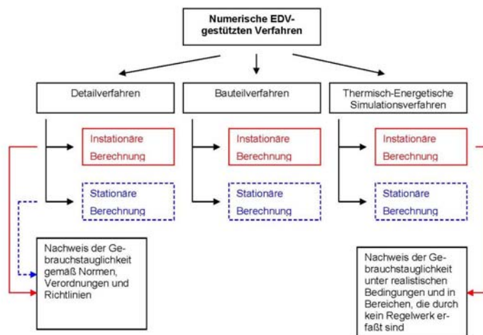
Diagramm 2: Einteilung der numerischen Verfahren zur Untersuchung der klimatischen Verhältnisse in Wohnmobilen
